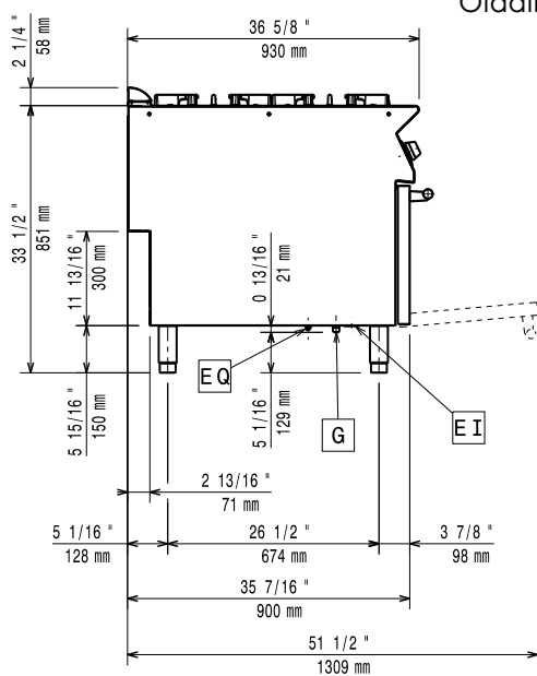
Oldalnézet
